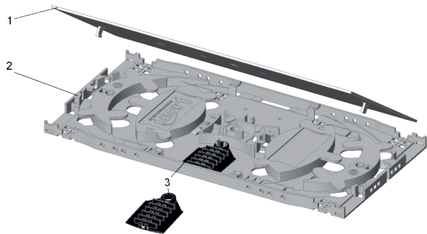
Panoramica scatola di giunzione conduttore in fibra ottica 1=copertura, 2=scatola di giunzione, 3=supporto protettore giunzione 6 vie
