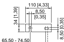
Escuadra de fijación de pared montada en raíl de montaje DIN
