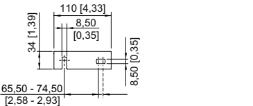
Escuadra de fijación de pared montada en raíl de montaje DIN
