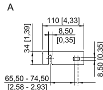
Escuadra de fijación de pared montada en riel de montaje DIN
