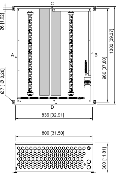
1 x BusRail 16 ranuras conexión
