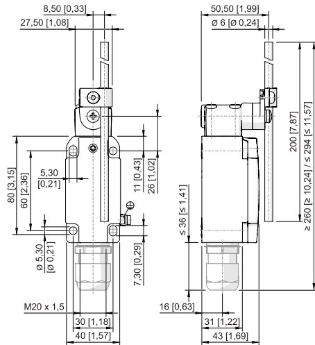
Palanca de varilla 8074/2.-DD-40
