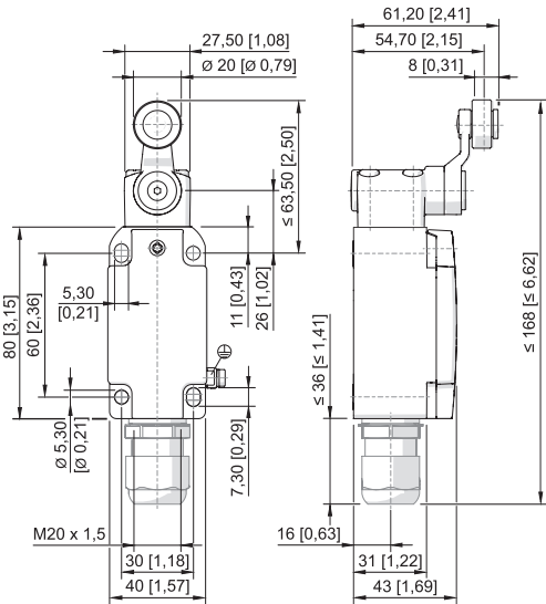
Palanca giratoria 8074/2--D-40
