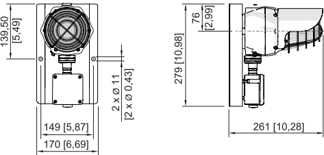
Esquema de medida (todas las medidas en [pulgadas]) – Se reserva el derecho a modificaciones
