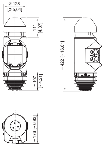
Bocina omnidireccional YL60/3
