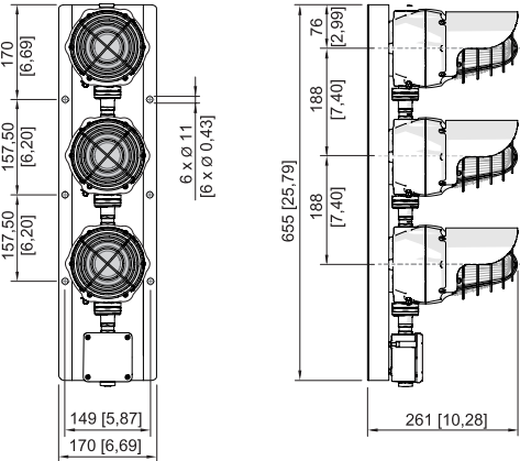
Esquema de medida (todas las medidas en [pulgadas]) – Se reserva el derecho a modificaciones
