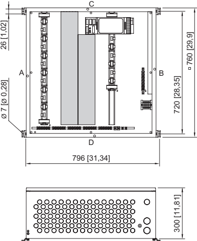
Esquema de medida (todas las medidas en [pulgadas]) – Se reserva el derecho a modificaciones
