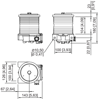
Esquema de medida (todas las medidas en [pulgadas]) – Se reserva el derecho a modificaciones
