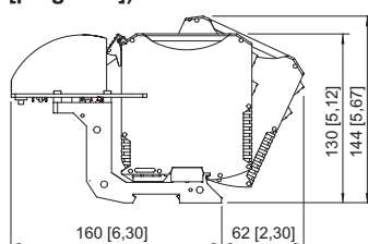
9419 Soporte bus con módulos
