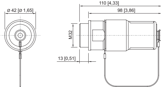
Base de brida Ex e 8595/1
