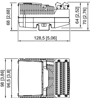
Esquema de medida (todas las medidas en [pulgadas]) – Se reserva el derecho a modificaciones
