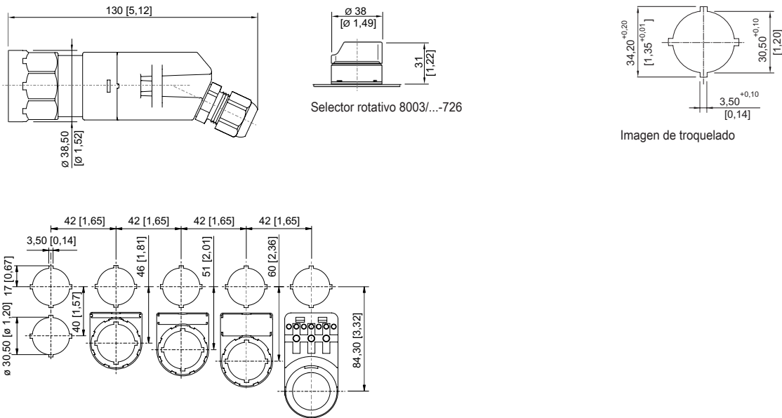
Dimensiones de montaje con/sin placa de identificación adicional
