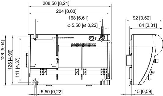
Esquema de medida (todas las medidas en [pulgadas]) – Se reserva el derecho a modificaciones
