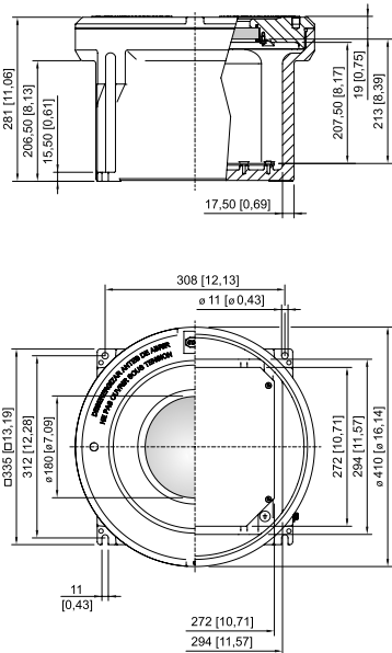
Tamaño de envolvente 6 con ventana
