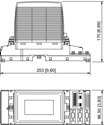
CPU y fuente de alimentación para zona 1 con conexión a través de terminales Ex e
