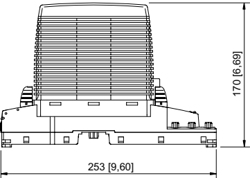
CPU y fuente de alimentación para zona 1 con conexión mediante extremo libre del cable
