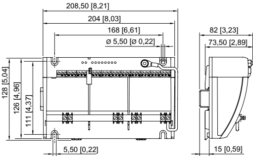
Acoplamiento de dispositivo de campo, 8 pistas, sin envoltorio
