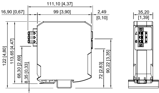
Esquema de medida (todas las medidas en [pulgadas]) – Se reserva el derecho a modificaciones
