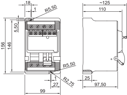
Interruptor diferencial, de 4 polos, 8562/54-...
