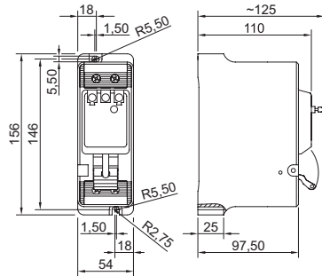
Interruptor diferencial, de 2 polos, 8562/52-...
