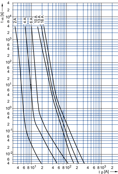
Curva característica tiempo/corriente de los insertos de molde (margen de tolerancia máx. ± 10 %)
