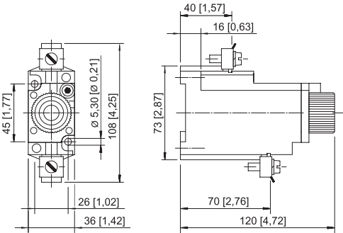
Elemento fusible 8561/01
