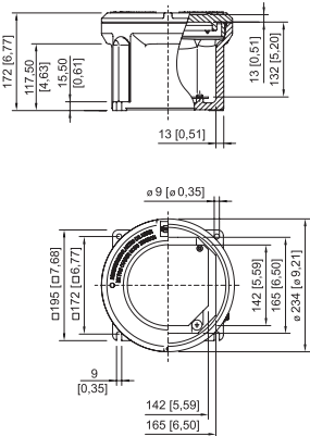
Tamaño de envolvente 3 sin mirilla
