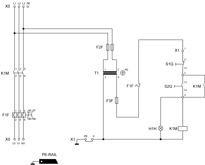
Esquema de circuito
