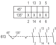
Esquema de conmutación 8008/2-613
