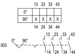
Esquema de conmutación 8006/4-003-00
