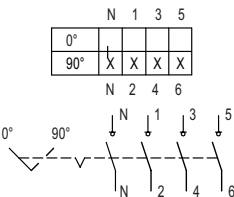
Esquema de conmutación 8544/1-4 and 8549/1-4
