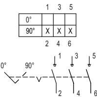
Esquema de conmutación 8544/1-3 and 8549/1-3
