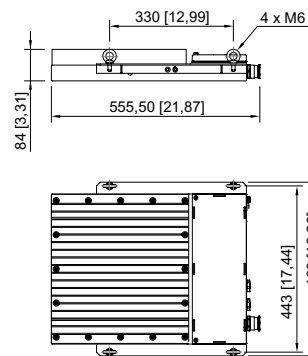
Proyector con disipador térmico, con cáncamos
