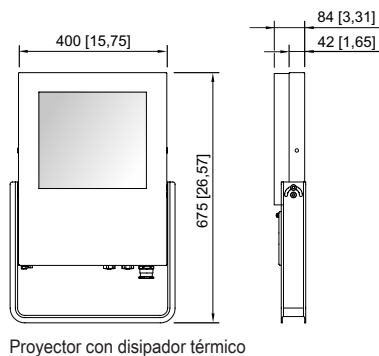
Proyector con disipador térmico
