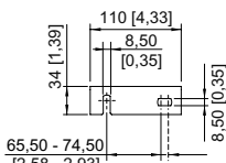
Escuadra de fijación de pared montada en riel de montaje DIN
