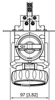
Base de brida de 4 polos Posición horaria 9 h, 10 h, 11 h
