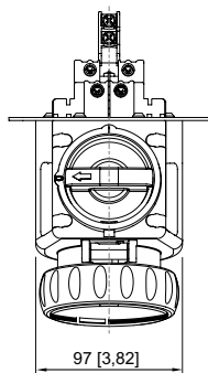
Base de brida de 5 polos Posición horaria 5 h, 6 h, 7 h
