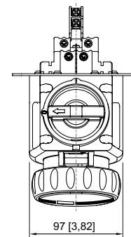
Base de brida de 5 polos Posición horaria 9 h, 10 h, 11 h
