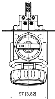
Base de brida de 4 polos Posición horaria 5 h, 6 h, 7 h
