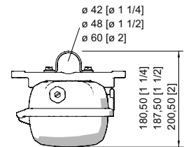
Collier de serrage monté sur support rail DIN
