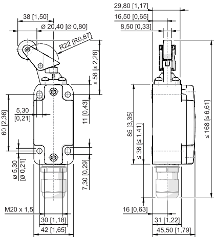
Levier à galet 8070/2-3-WPH-U60
