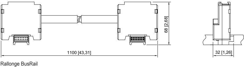
Plan d'encombrement (toutes les dimensions sont en mm [pouces]) – sous réserve de modifications
