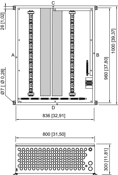
Plan d'encombrement (toutes les dimensions sont en mm [pouces]) – sous réserve de modifications
