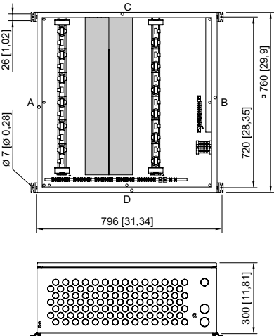
1 x BusRail pour 12 emplacements
