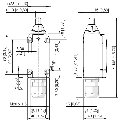
Poussoir à calotte sphérique 8074/2-.-W-40
