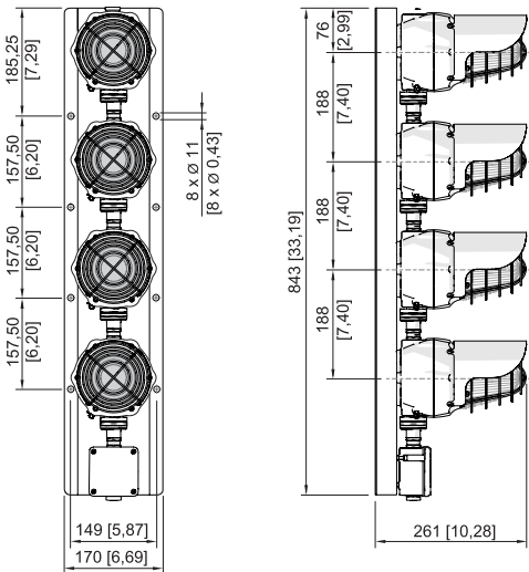
Plan d'encombrement (toutes les dimensions sont en mm [pouces]) – sous réserve de modifications
