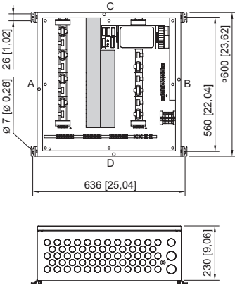
Plan d'encombrement (toutes les dimensions sont en mm [pouces]) – sous réserve de modifications
