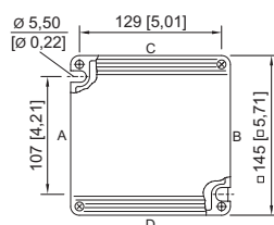
8118/3. Boîtier taille 3
