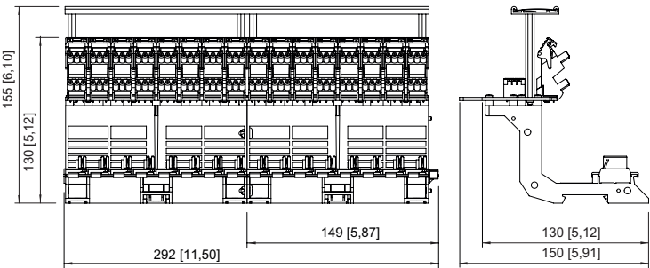
Type 9195/16-....., 16 emplacements
