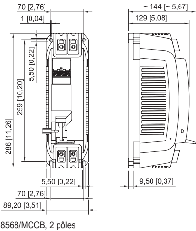
Plan d'encombrement (toutes les dimensions sont en mm [pouces]) – sous réserve de modifications
