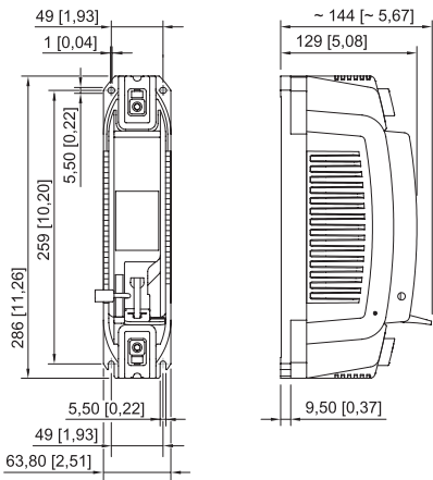
8568/MCCB, 1 pôle
