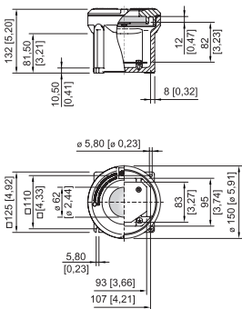
Boîtier taille 1 avec hublot
