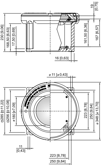
Boîtier taille 5 avec hublot
