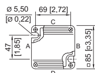
8118/1. Boîtier taille 1
