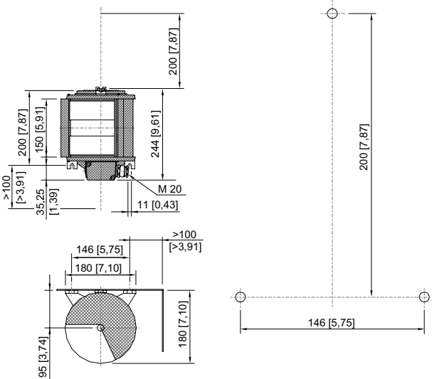
TEF 2850 Lanterne de secteur
